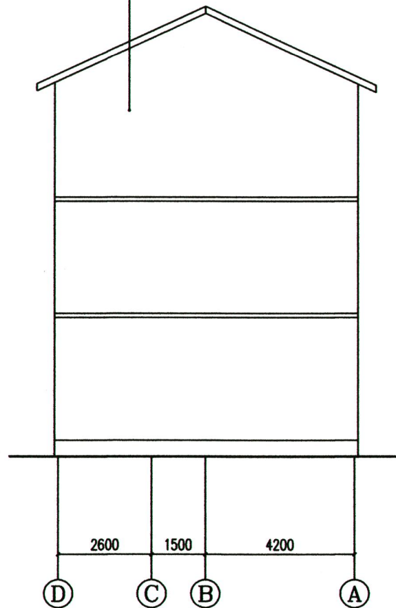
左立面图 1:100
