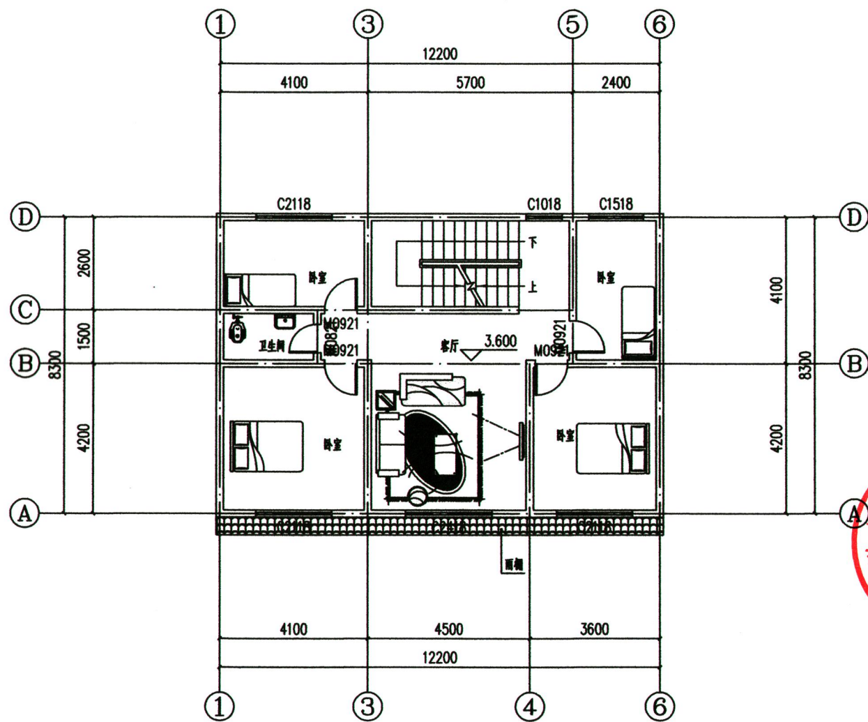
二层平面图 1:100
