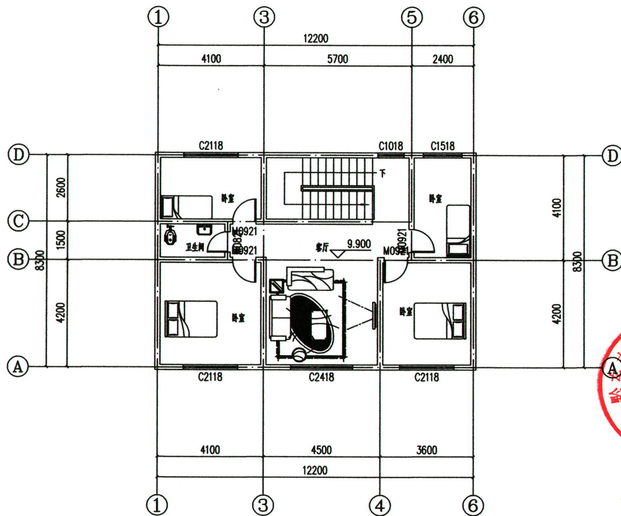
三层平面图 1:100
