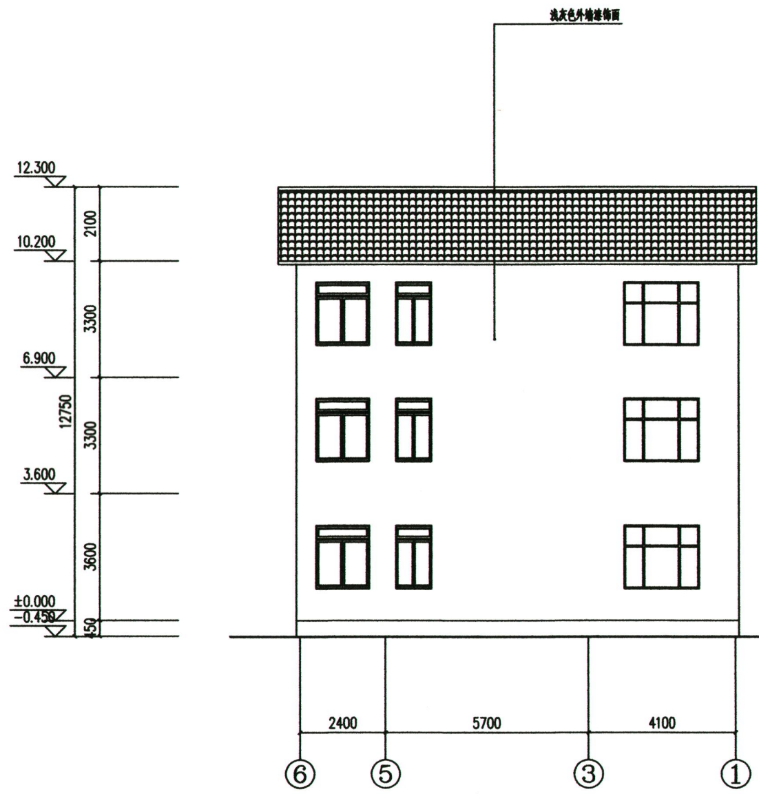
背立面图 1:100
