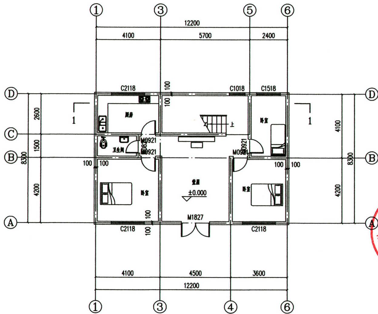
一层平面图 1:100
