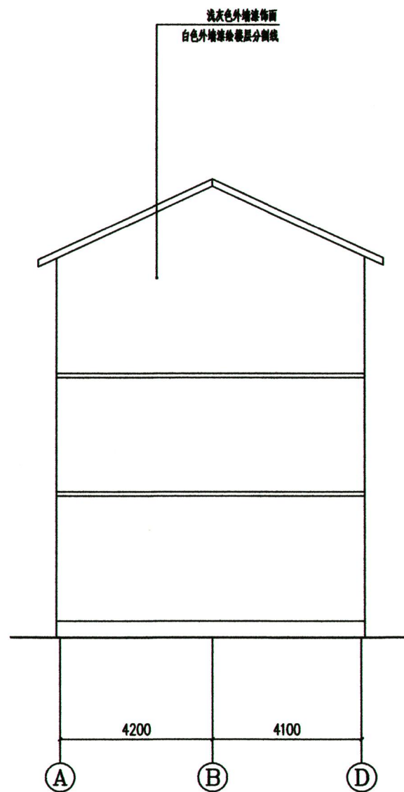
右立面图 1:100
