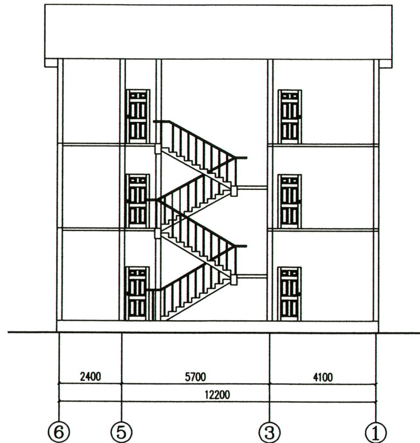
1-1剖面图 1:100
