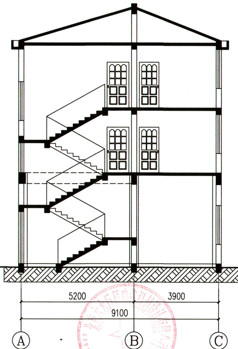
1~1剖面图 1:100
