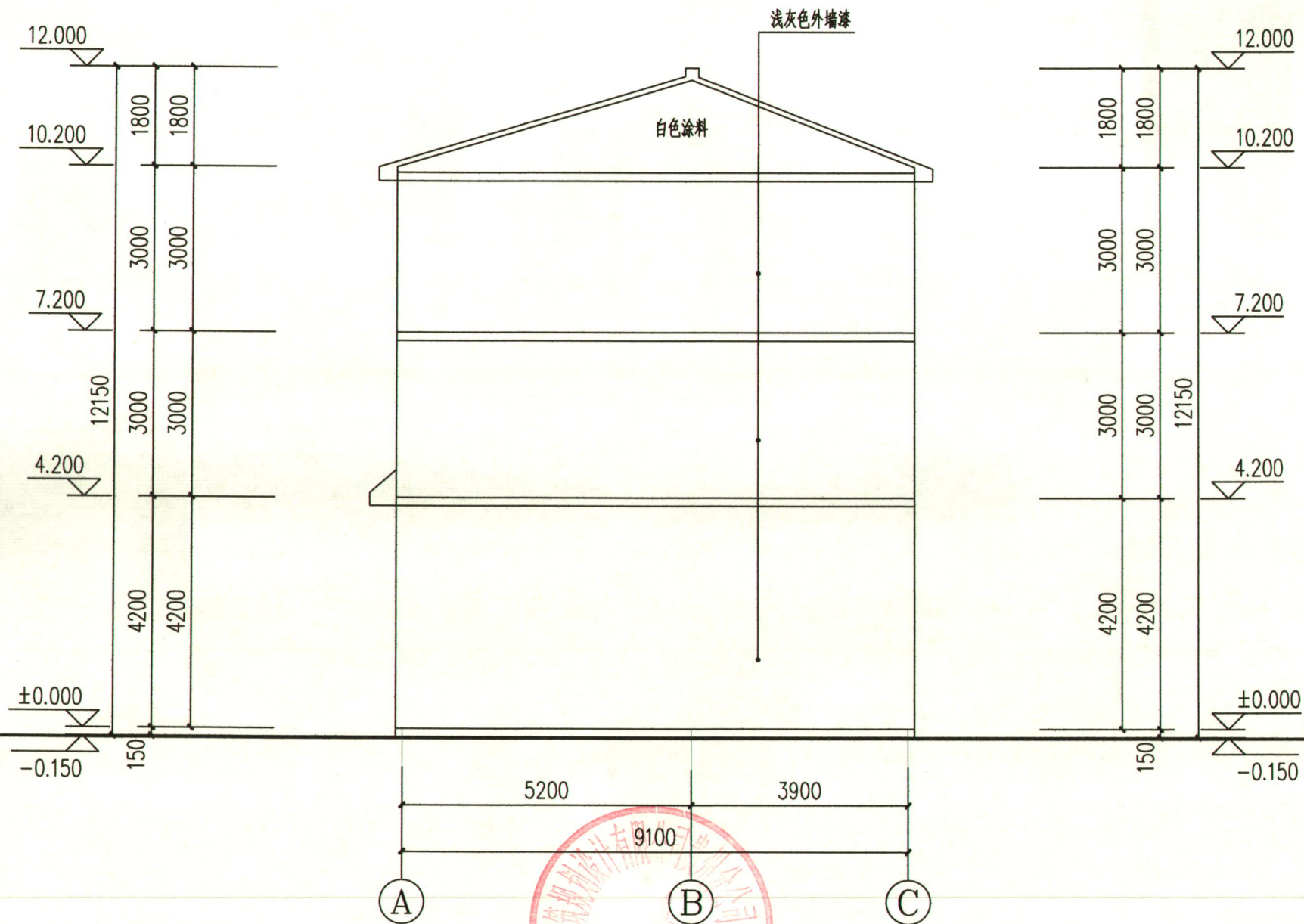
Ⓐ ~ Ⓒ 立面图 1:100
