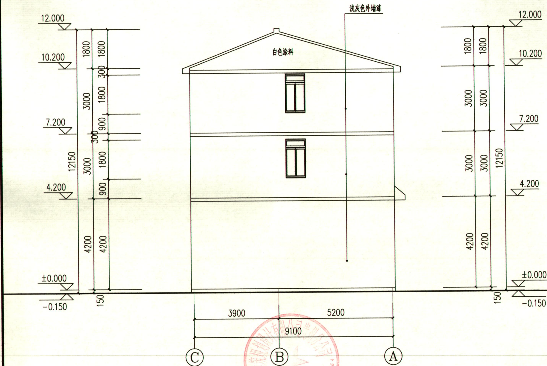
C~A立面图 1:100
